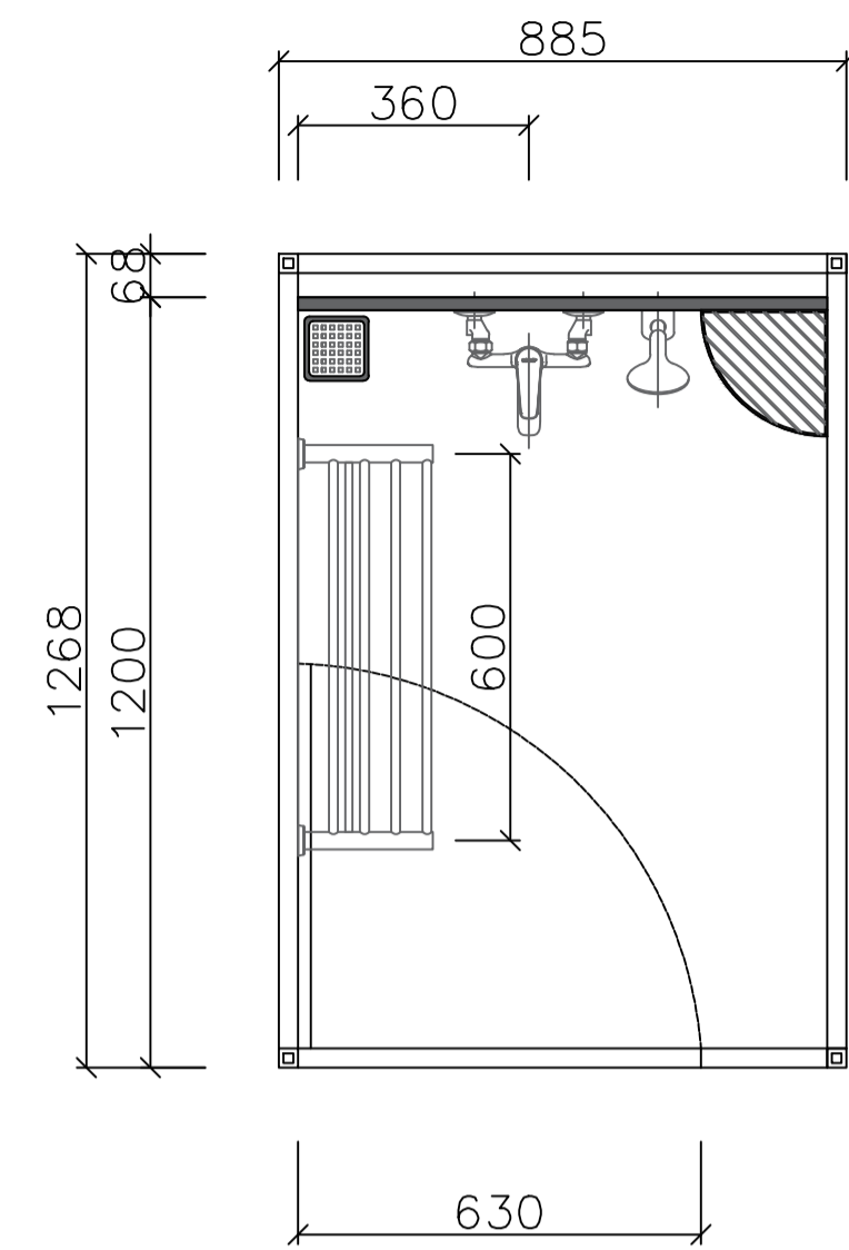
平面配置圖
