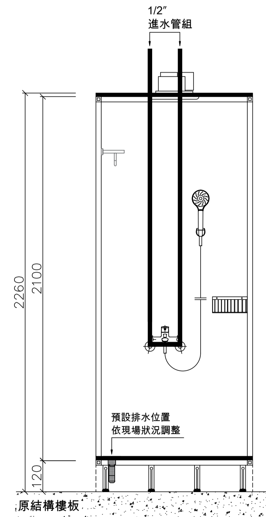
進水及排水正立面圖
