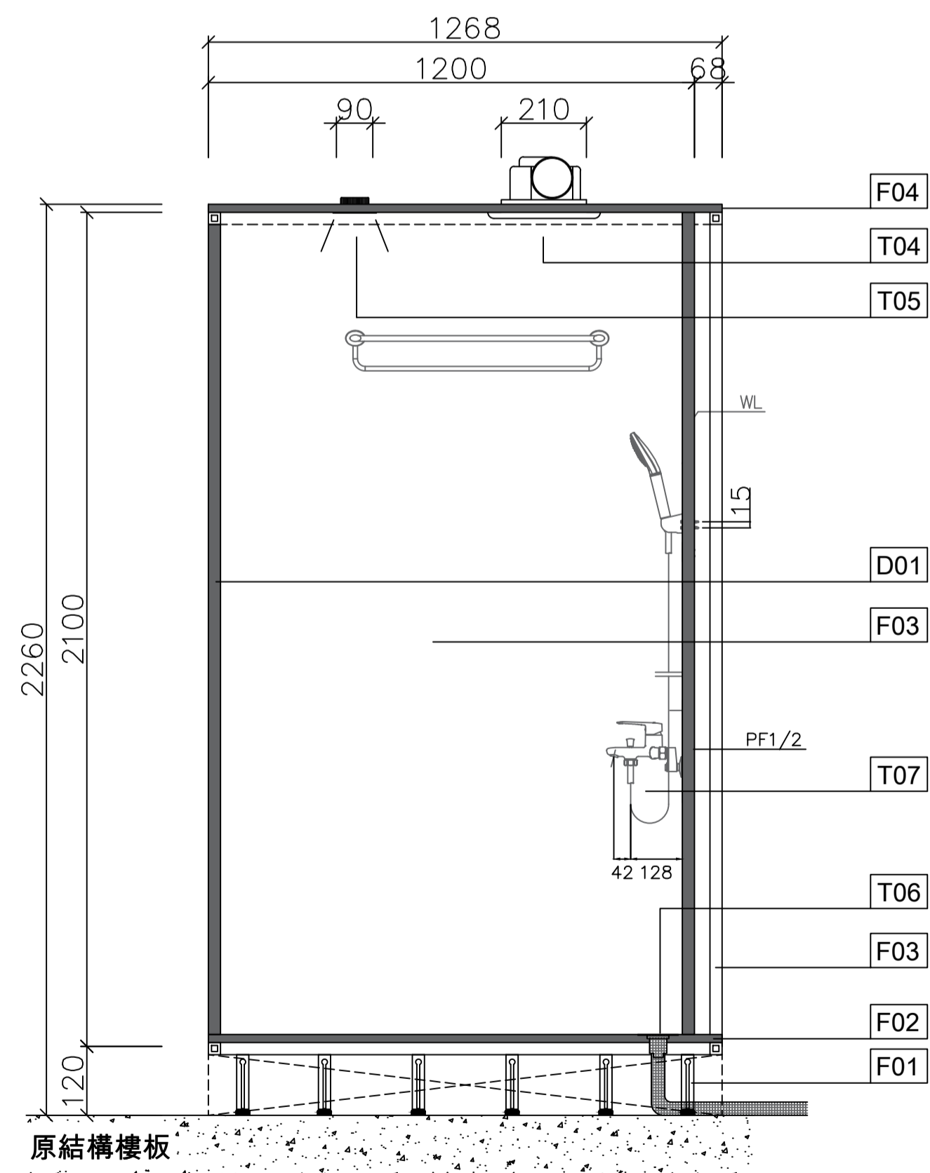
側立面配置圖
