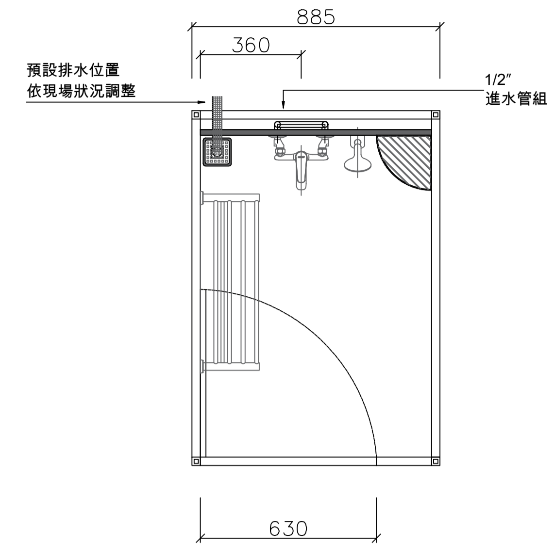
進水及排水平面圖
