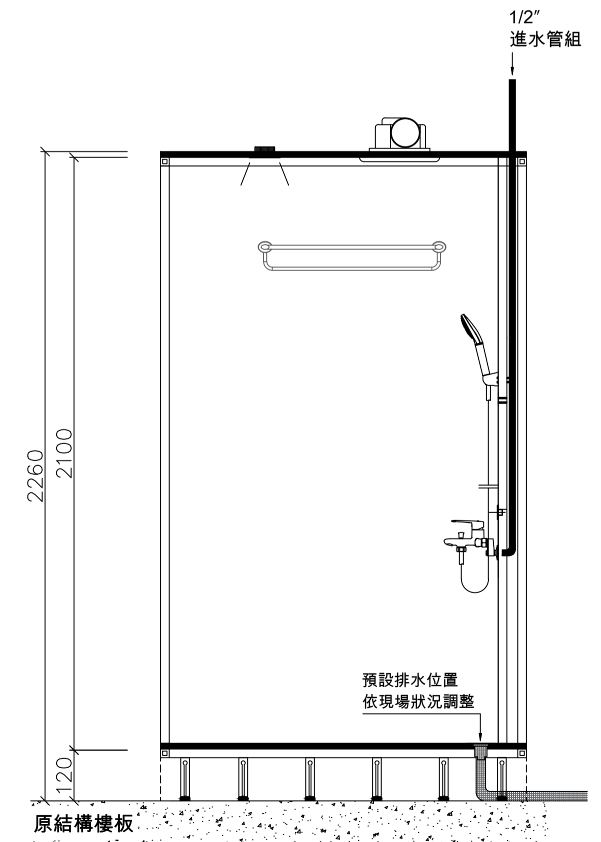
進水及排水側立面圖
