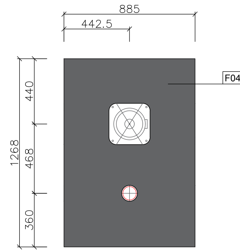
天花板配置圖
